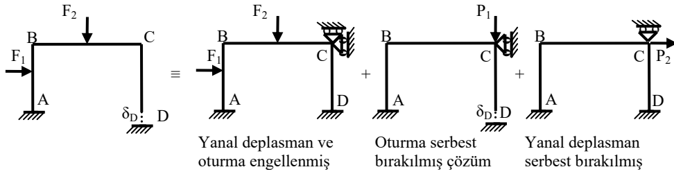
Şekil 2. Yanal deplasman ve oturma görülen çerçevenin çözümü
